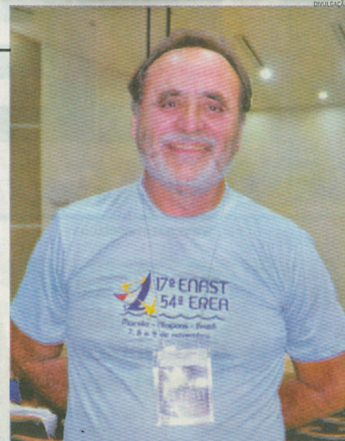
AUGUSTO DAMINI, astrofísico brasileiro de renome internacional, visitou Maceió para proferir a palestra de abertura do 17º Encontro Nacional de Astronomia, realizado sob a organização da Universidade Federal de Alagoas.
